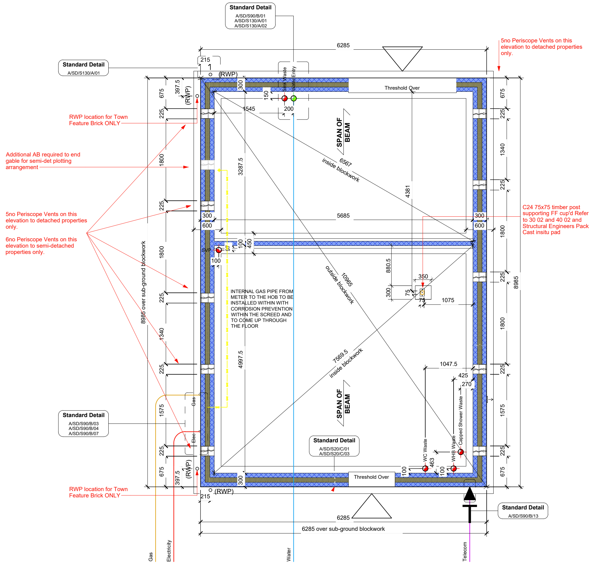
1 Foundation 1-50 1 : 50
